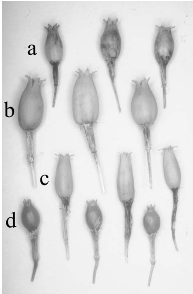
Fig. 2. Capsule shape – a: Silene saxifraga ; b: S. notarisi ; c: S. multicaulis ; d: S. hayekiana . – Vouchers: a: M. Nerone, Il Cimaio, Gubellini (PESA); b: M.ti Sibillini, dintorni di Bolognola, Gubellini (PESA); c: M.ti Sibillini, Valle del Fargno, Gubellini (PESA); d: Val di Fassa, Gruppo del Catinaccio, Val d'Udai, Brilli-Cattarini (PESA).
